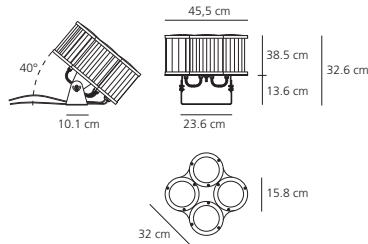
Metaponto HALO 3x150W (B 15d) – ES
