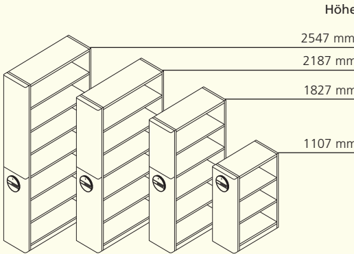
Erhältliche Regalbreiten 1200 mm, 1000 mm, 900 mm, 800 mm, 600 mm
