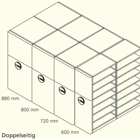
Doppelseitig
