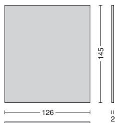
Anta scorrevole per 3 vani, fronte vetro laccato Sliding door for 3 spaces, with lacquered glass Schiebetür für 3 Räume, mit Vorderstück aus lackiertem Glas
