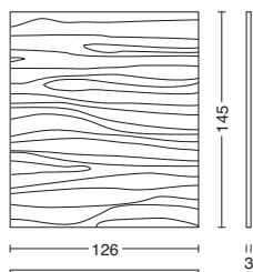
Anta scorrevole per 3 vani, fronte legno Sliding door for 3 spaces, with wooden front Schiebetür für 3 Räume, mit Holz Vorderstück
