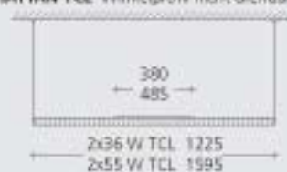
MANHATTAN TCL Winkelprofil nicht drehbar
